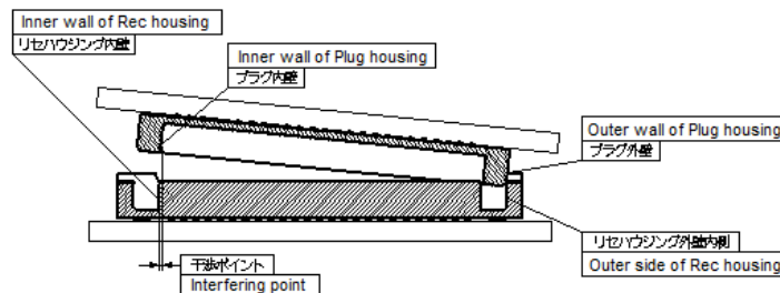
× 図-3 外壁合せによる嵌合 (Not Good) Figure-3 Mating aligning to outer wall of housings (Not Good)
