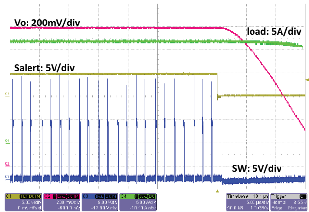
Fig. 15 - SiC453 OCP
